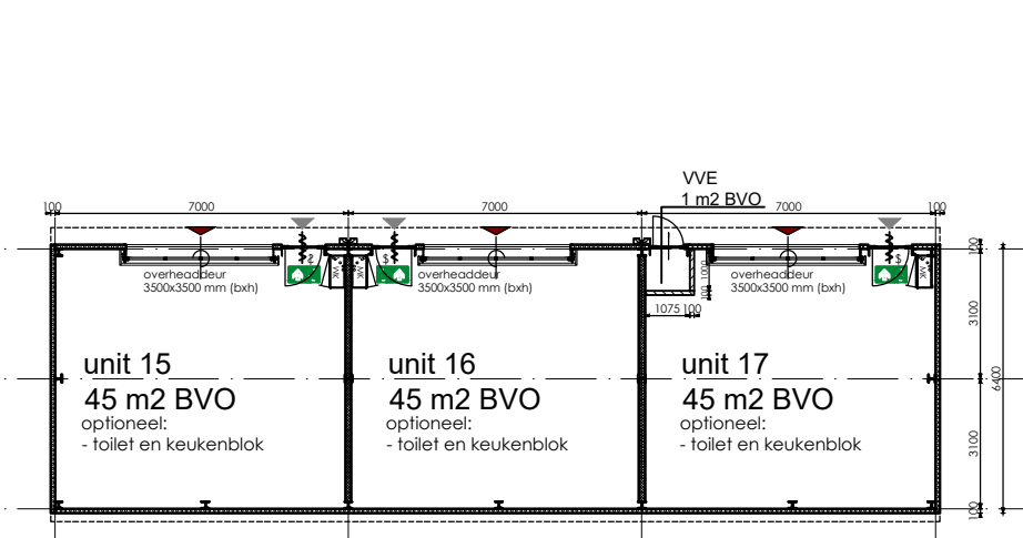
Begane grond BLOK 2 Peil=0
