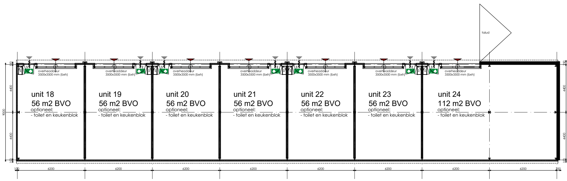
Begane grond BLOK 3 Peil=0
