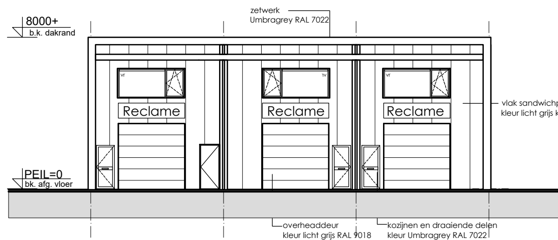
Voorgevel Blok 2
