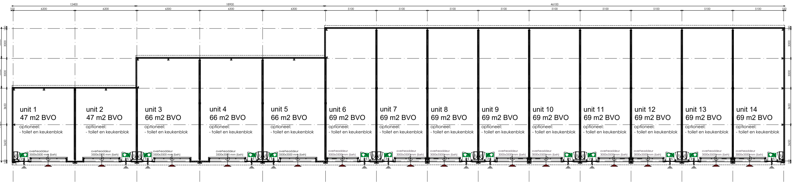
Begane grond BLOK 1 Peil=0
