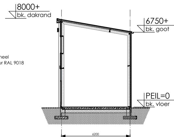
Doorsnede Blok 2
