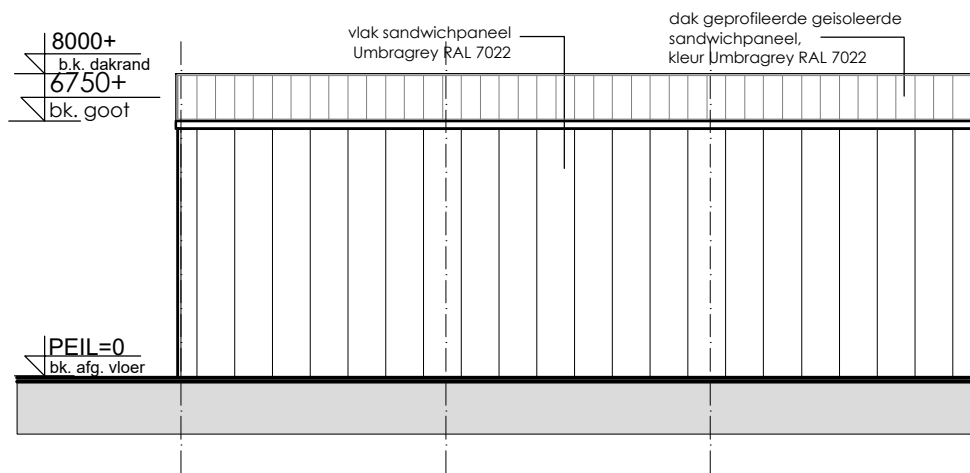
Achtergevel Blok 2
