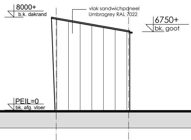
Rechter zijgevel Blok 2 (linker zijgevel gespiegeld)
