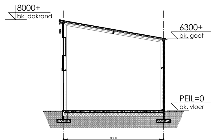
Doorsnede Blok 3
